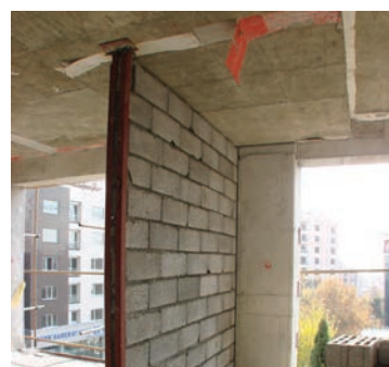
مهاری بندی لیه انتهایی دیوار با دهانه آزاد بیش از ۱/۵ متر
