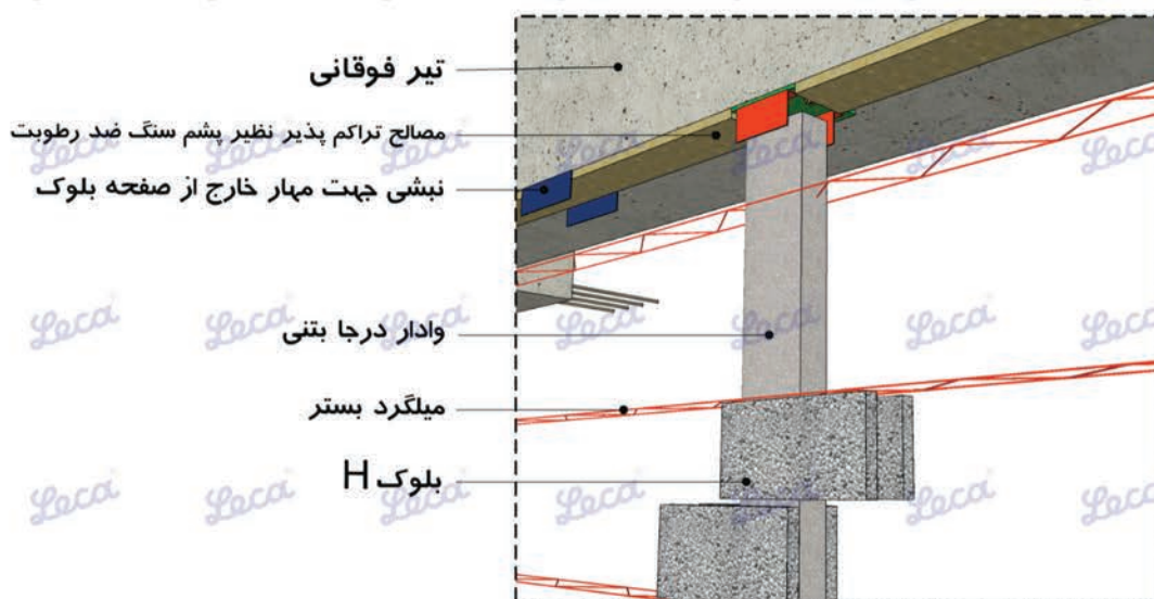
نحوه اتصال وادار بتنی به زیر تیر
