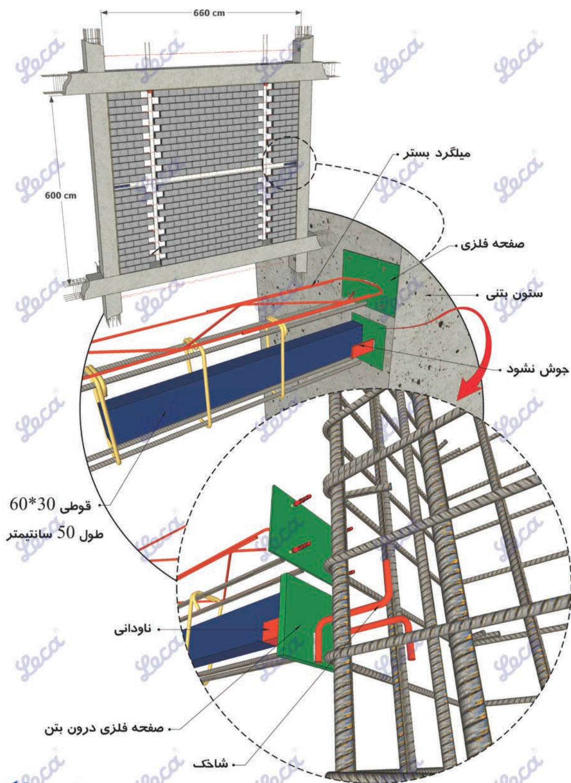
جزئیات اتصال وادار افقی به ستون بتنی
