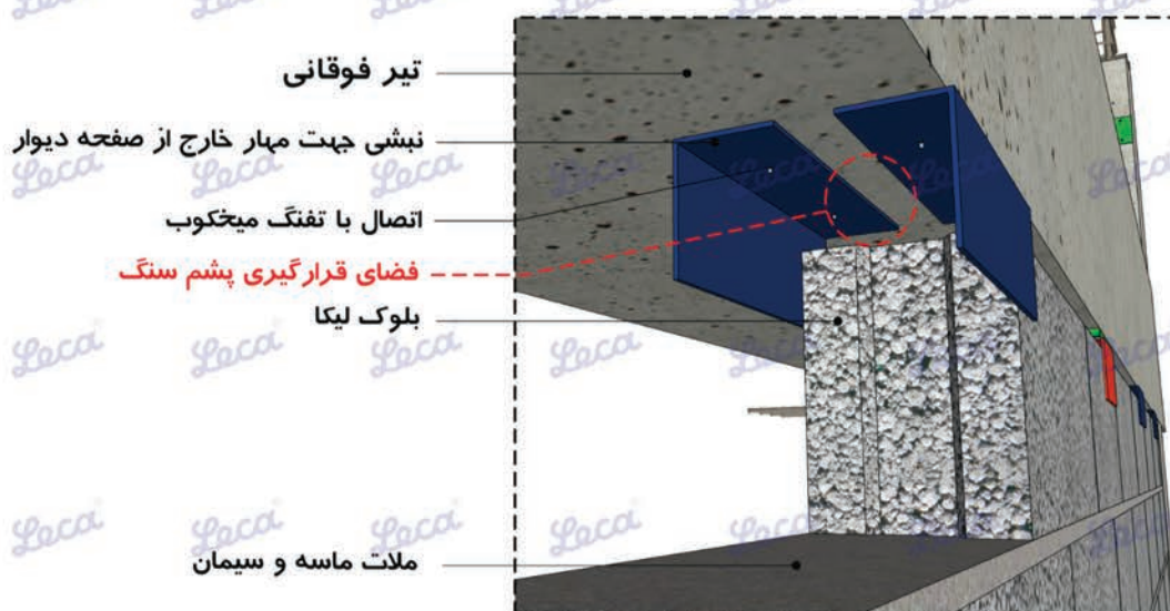
نحوه مهار آخرین رج دیوار
