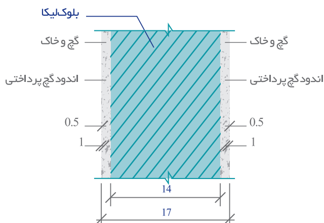
شکل ۲: جزئیات دیوار ساخته شده با بلوک بتن سبک لیکا، دو طرف اندود
