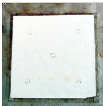
شکل ۷- سطح غیر معرض آزمون در حین آزمون
