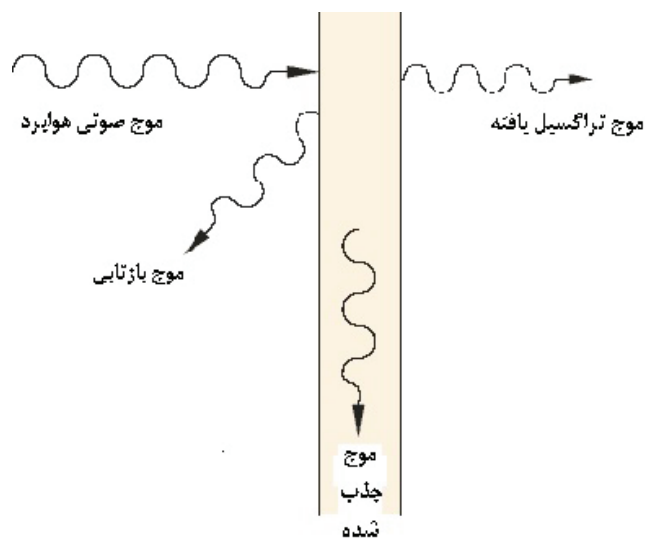
تراگیسل صدای هوابرد از طریق یک جداکننده
