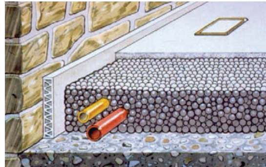
عبور لوله ها از درون لایه کفسازی
